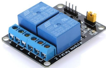
Fig: Relay Module
