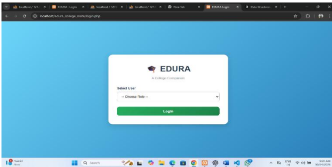
Fig 10.1.1 Login-page
